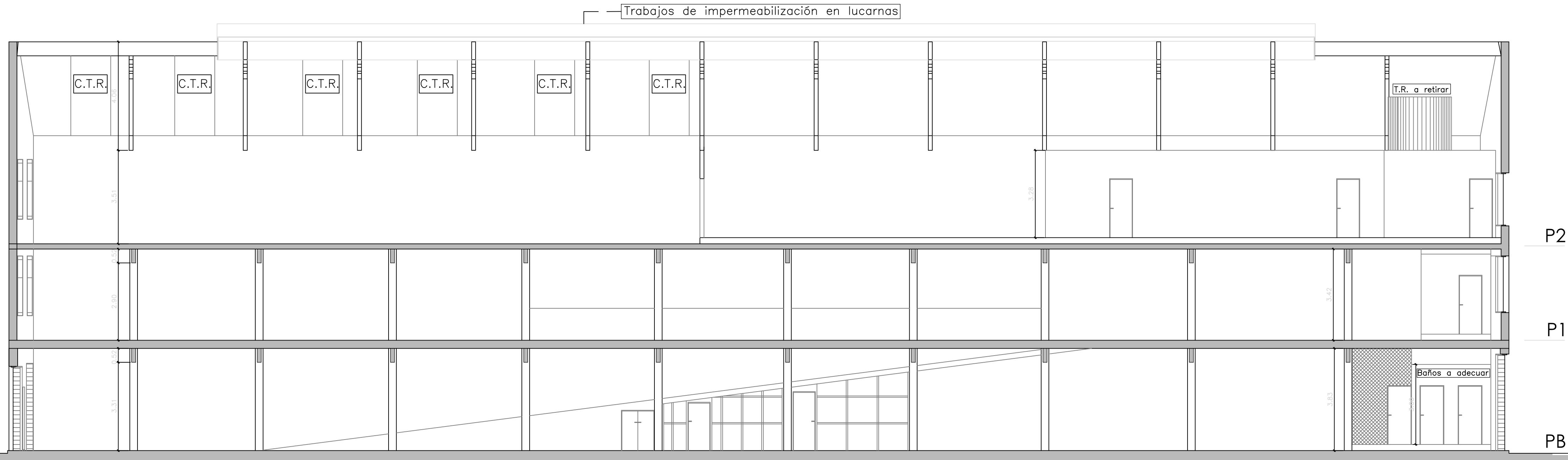
Corte B - B' AV. BELGRANO 2252 - Anexo aulas y taller UNA
