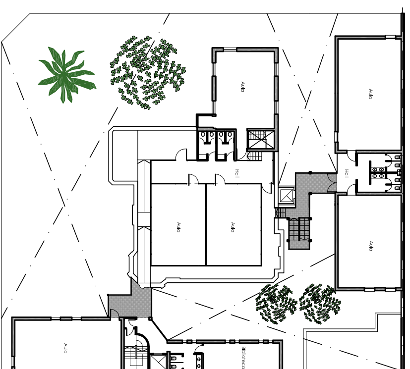
PLANTA 3º PISO
