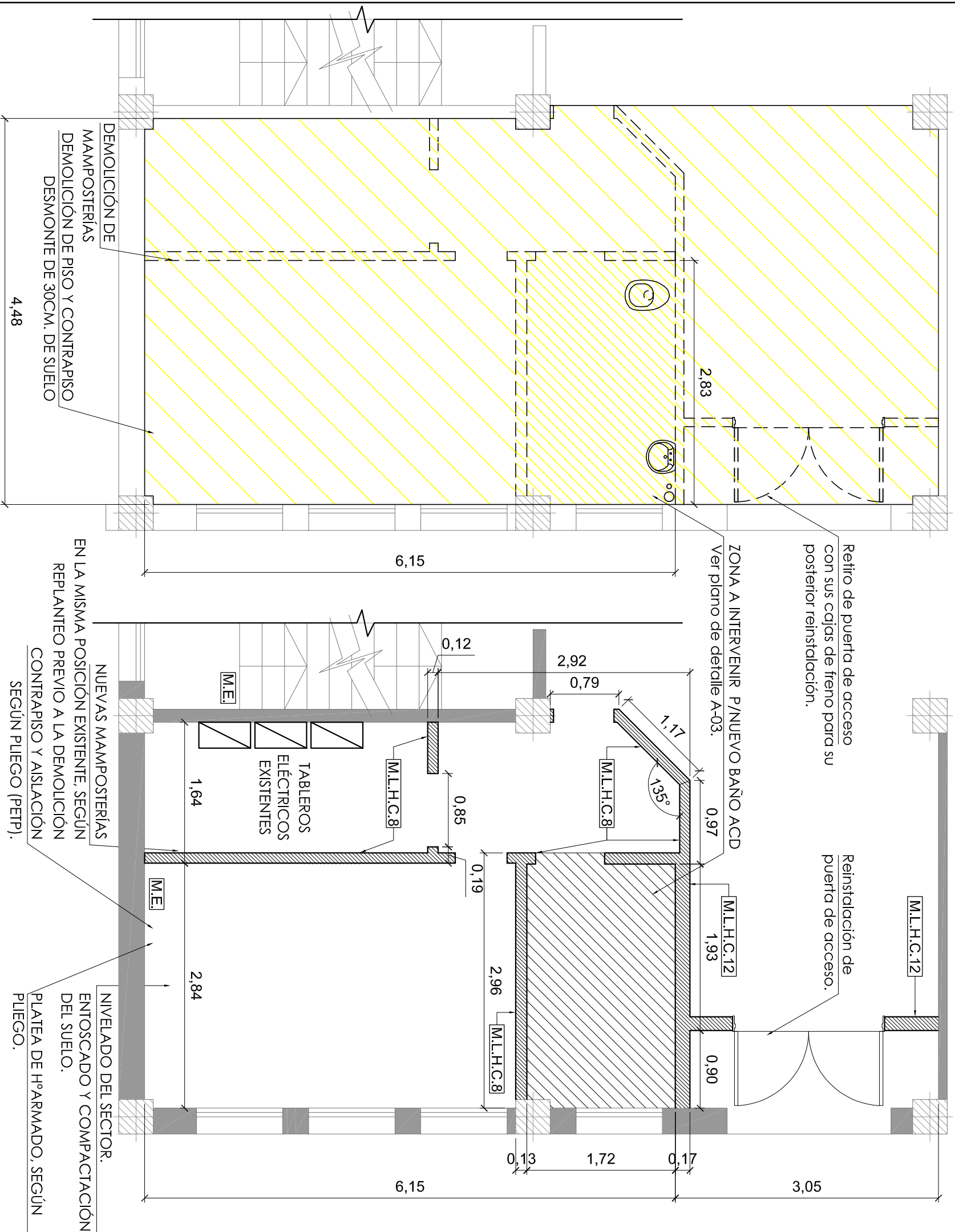
PLANTA DEMOLICIÓN EXISTENTE ESC. 1:50
