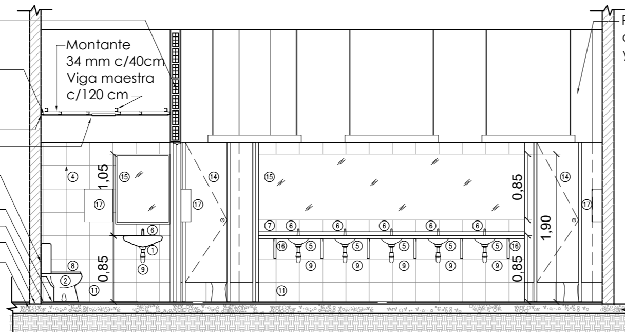
CORTE 3 - ESC. 1:50
