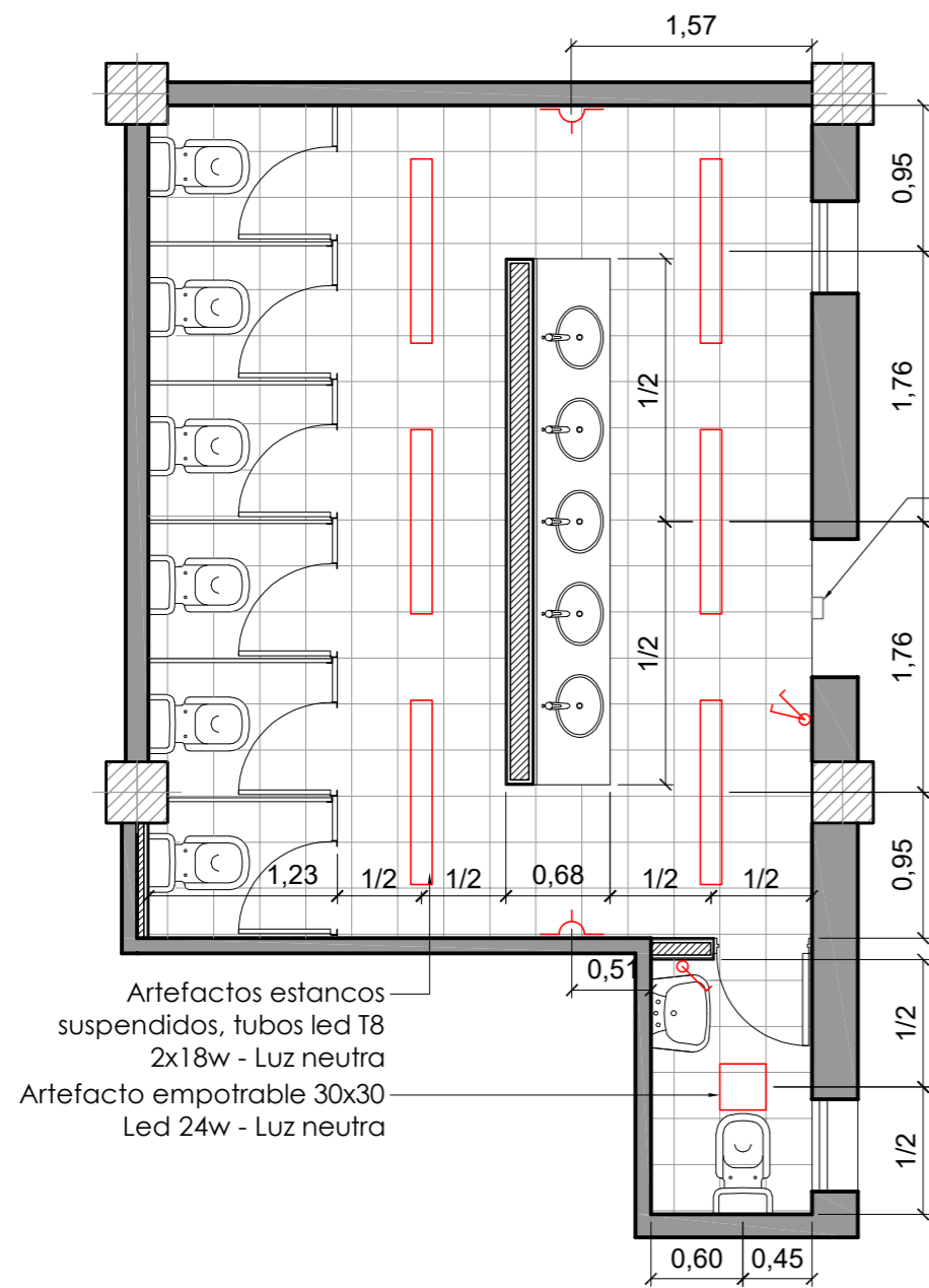
INSTALACIÓN ELÉCTRICA ESC. 1:50
