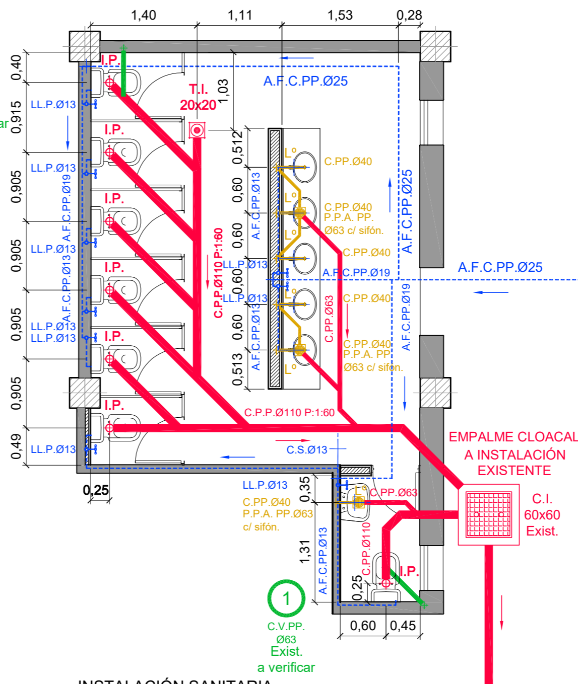
INSTALACIÓN SANITARIA ESC. 1:50
